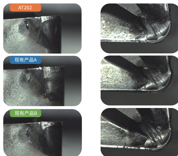
切削时间 18.4 分钟对比
